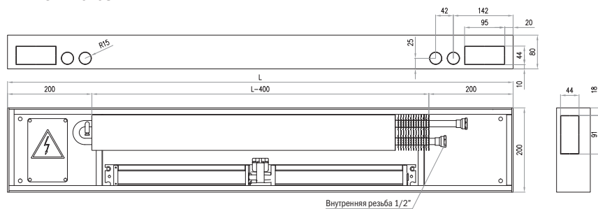
ТКВ-13 Lx20x08
