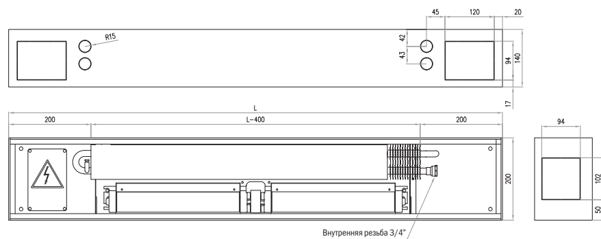
ТКВ-13 Lx20x14
