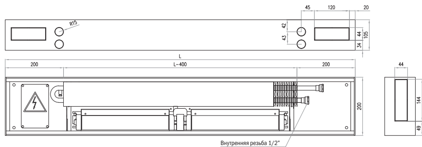
ТКВ-13 Lx20x10
